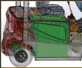
배터리 중앙 하단 배치
